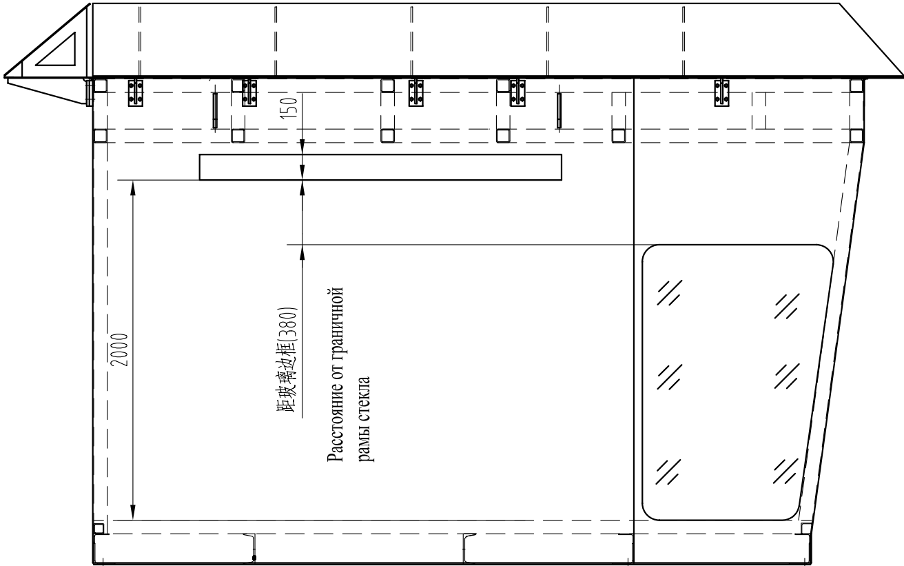
Чертеже монтажа настенного электрорадиатора 壁挂式电暖气安装图
